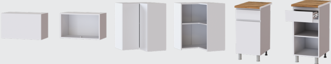
Окап 600 П6Х 600х360х318 Угловой навесной шкаф 600х600 угол прямой ПУВП 600х600х720х318 Рабочий стол с 1 ящиком 400 П4Р1 400х850х600
