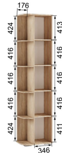
ЛШ-26 Шкаф торцевой 2212x350x544
