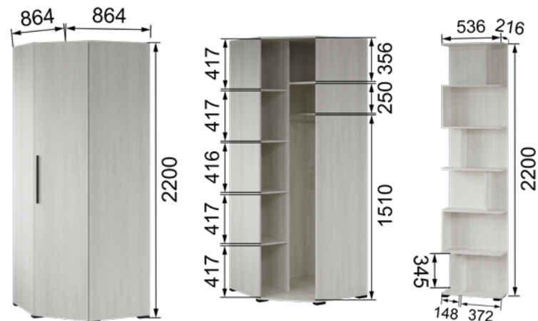
МШ-25 Шкаф угловой 2200x864x864
