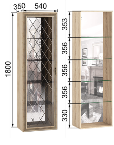
ЛШ-8 Пенал-витрина (надстраиваемый) 1800x540x350
