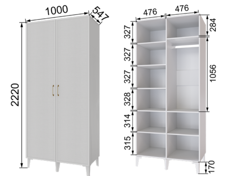
TШ-21 Шкаф двухстворчатый 2220x1000x547
