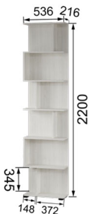
МШ-26 Угловой стеллаж 2200x216x536
