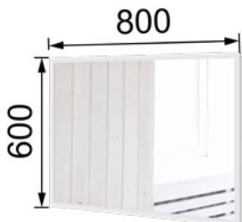
T3-20 Зеркало навесное 600x800/800x600x22
