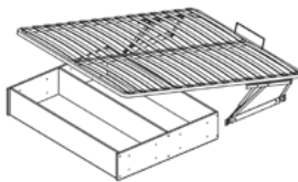
Ортопедическое основание с подъемным механизмом и ящиком для белья
