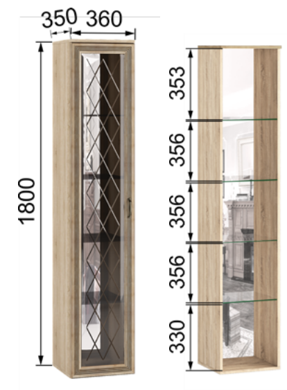
ЛШ-7 Пенал-витрина (надстраиваемый) 1800x360x350
