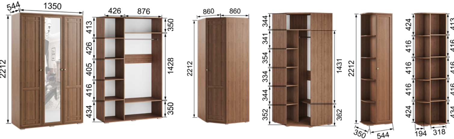
РШ-25 Шкаф трехстворчатый 2212x1350x544
