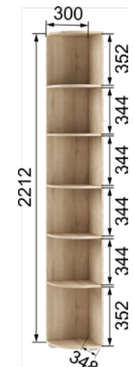
ЛШ-10 Угловой стеллаж 2212x300x348
