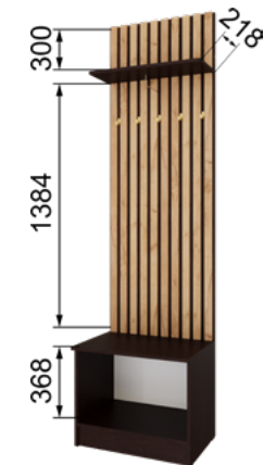
КПТВ-1 Тумба с вешалкой 600 2200x602x430
