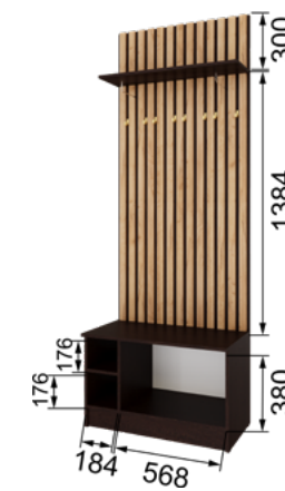
КПТВ-2 Тумба с вешалкой 800 2200x802x430
