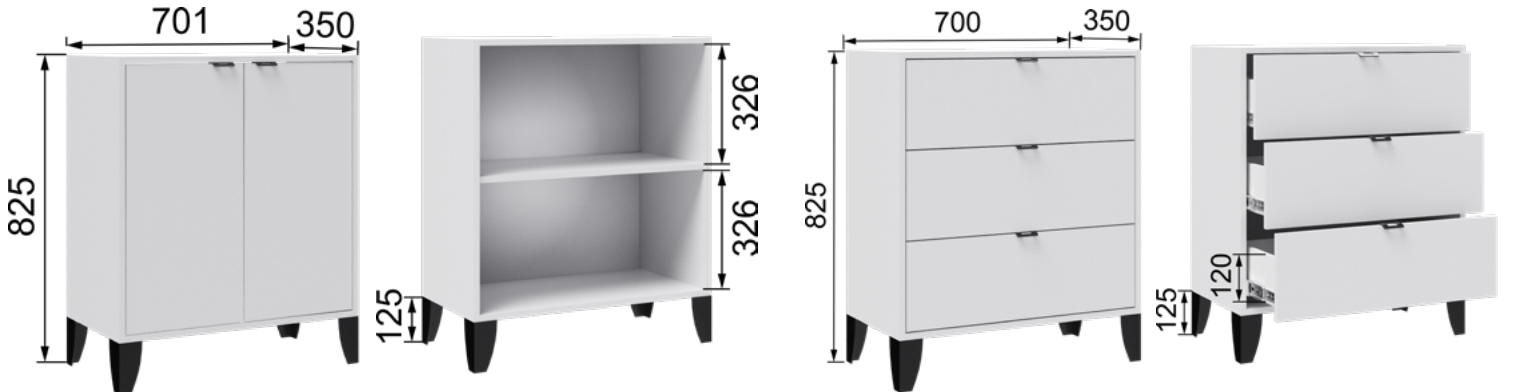
ГШ-2 Шкаф 825x700x350 ГК-1 Комод 825x700x350
