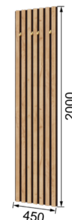
КПВ-1 Вешалка 450 2000x450x32
