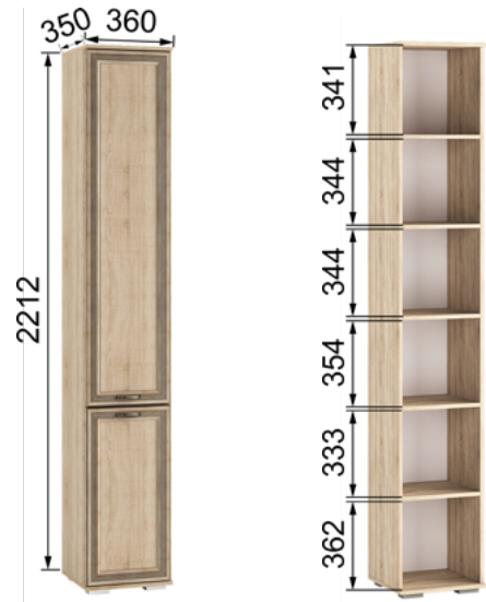
ЛШ-1 Пенал с полками 2212x360x350
