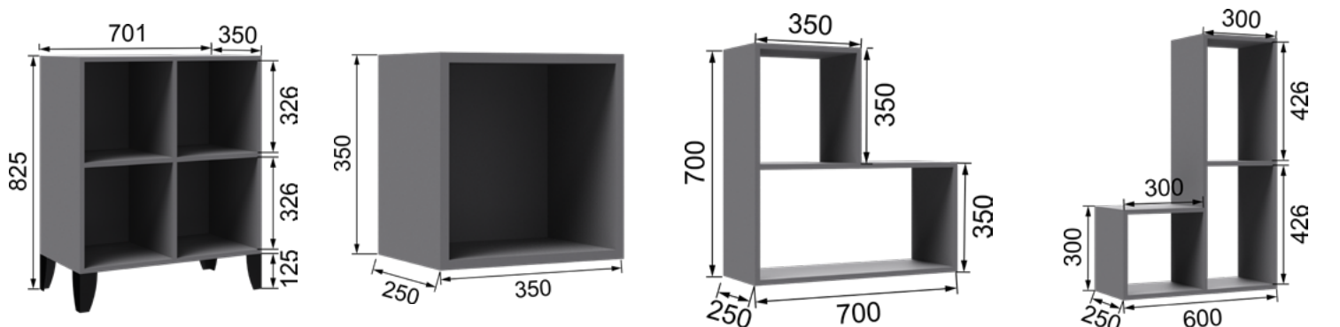
ГС-1 Стеллаж открытый 825x700x350 ГКБ-1 Куб 350x350x250 ГН-1 Полка 700x700x250 ГН-2 Полка 600x900x250
