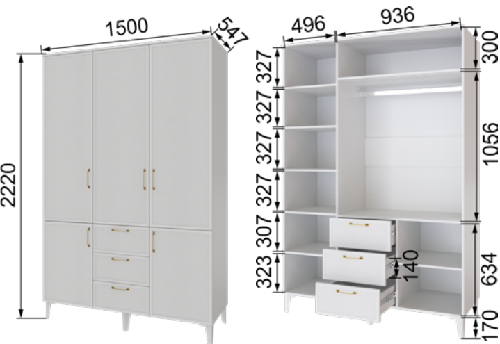
TШ-24 Шкаф трехстворчатый с ящиками 2220x1500x547
