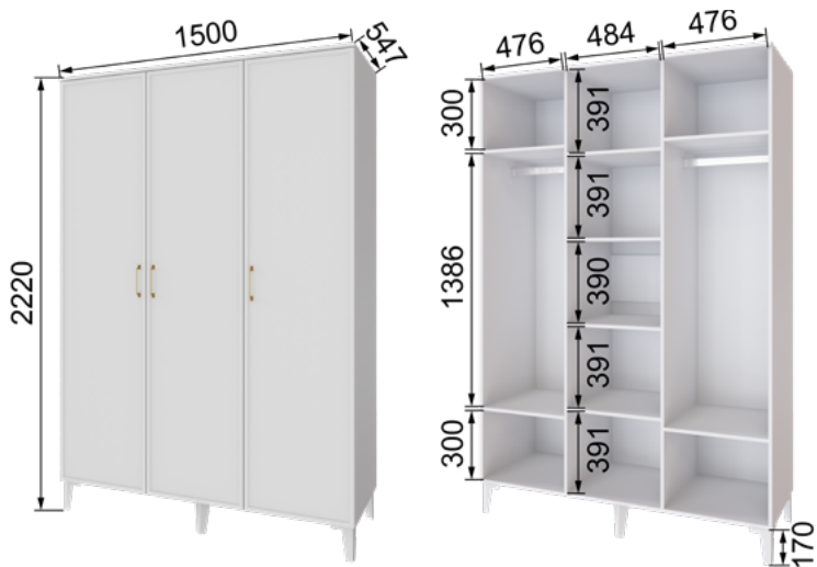
TШ-23 Шкаф трехстворчатый 2220x1500x547
