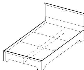
Кровать с настилом ЛДСП: КР-2_1,6 1770x970x2070 (под матрас 1600x2000) КР-2_1,4 1570x970x2070 (под матрас 1400x2000) КР-2_1,2 1370x970x2070 (под матрас 1200x2000)
