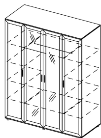
ШК-4 1600x2126x545
