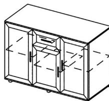
ТБ-3 1200x866x445
