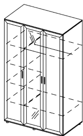
ШК-3 1200x2126x545
