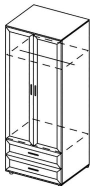
ШЯ 800x2126x545
