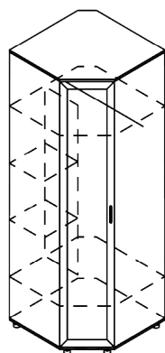
Ш-УГ-М 720x2126x720
