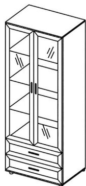
ШЯ-С 800x2126x445
