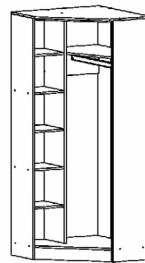
ПРН.13 Шкаф угловой (850x2064x850)
