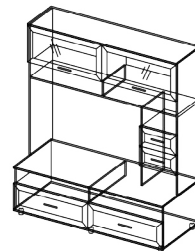
WM-4 1600x1930x545 (под ТВ 1184x836)
