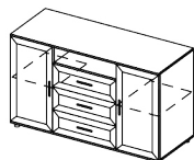
ТУ 1400x866x445
