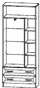
ПРН.11 Шкаф (800x2064x390)
