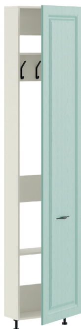
ПХН-554_Н8 (554 x 2233 x 220 мм)
