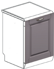
ПМ-450 (446 x 716 x 16 мм) ПМ-600 (596 x 716 x 16 мм)
