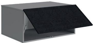
ГП-600_Н384 (600 x 384 x 572 мм) ГП-800_Н384 (800 x 384 x 572 мм)
