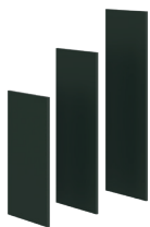
Фальшпанель к Шкафу_Н6 (626 x 309 x 16 мм) Фальшпанель к Шкафу_Н8 (818 x 309 x 16 мм) Фальшпанель к Шкафу_Н10 (1010 x 309 x 16 мм)
